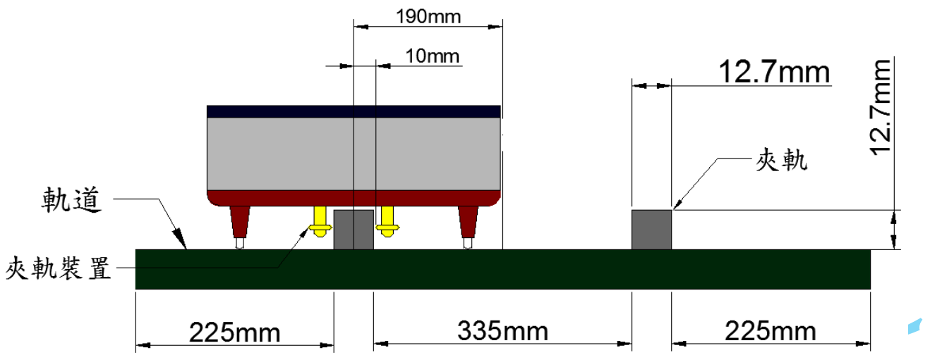
圖 6 軌道示意圖
